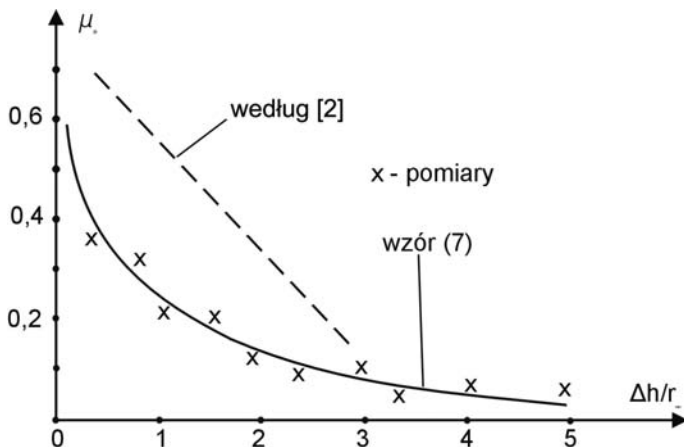
Rys. 3. Zmienność współczynnika wydatku przelewu szybowego
