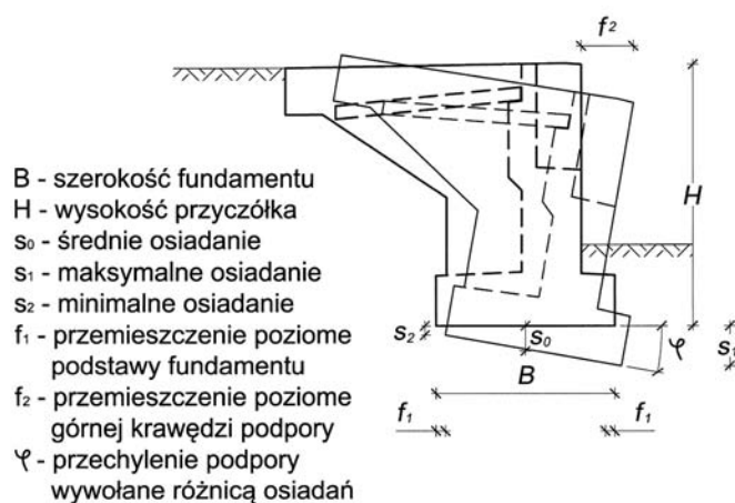
Rys. 1. Możliwe przemieszczenia przyczółka mostu [3]
