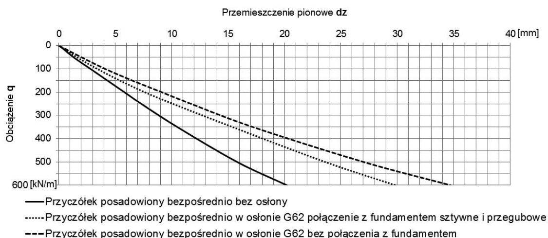
Rys. 8a. Przemieszczenie pionowe dz [mm] górnej krawędzi korpusu przyczółka w zależności od obciążenia przyłożonego w miejscu projektowanych łożysk w różnych przypadkach posadowienia bezpośredniego
