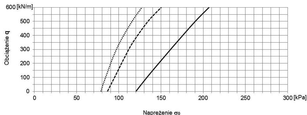
Rys. 8c. Napężenie w gruncie \sigma_1 [kPa] pod krawędzią przedniej odsadzki fundamentu przyczółka w zależności od obciążenia przyłożonego w miejscu projektowanych łożysk w różnych przypadkach posadowienia bezpośredniego
