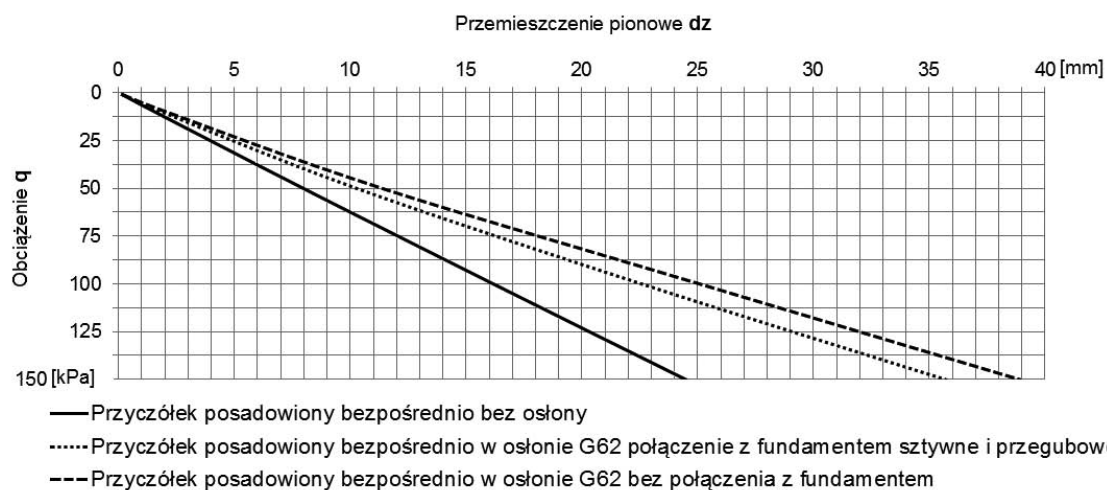
Rys. 9a. Przemieszczenie pionowe dz [mm] górnej krawędzi korpusu przyczółka w zależności od obciążenia naziomu w różnych przypadkach posadowienia bezpośredniego
