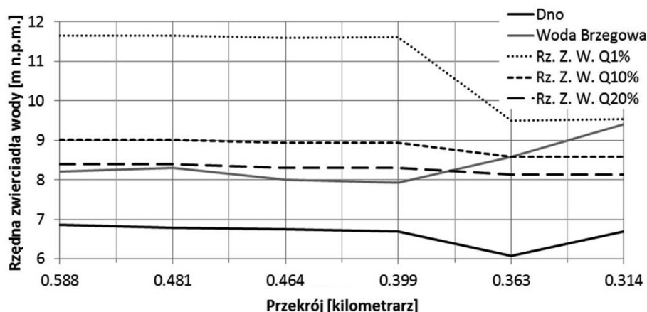
Rys. 10. Profil zwierciadła wody na odcinku Potoku Królewskiego przed przepustem pod nasypem kolejowym
