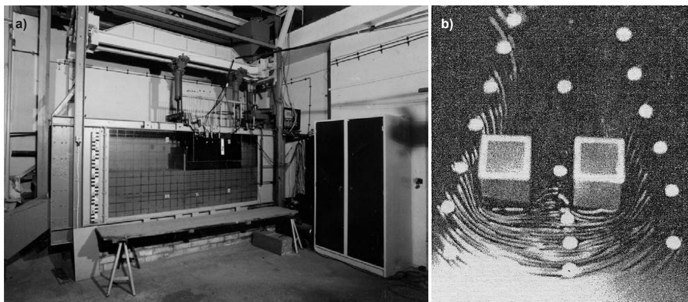
Rys. 2. Stanowisko w skali półtechnicznej z ekranem szklanym w Katedrze Geotechniki, Geologii i Budownictwa Morskiego WILiŚ PG do badania przemieszczeń modeli i deformacji podłoża gruntowego (a) oraz wynik rejestracji upłynięcia gruntu obciążającego pale (b) [7]
