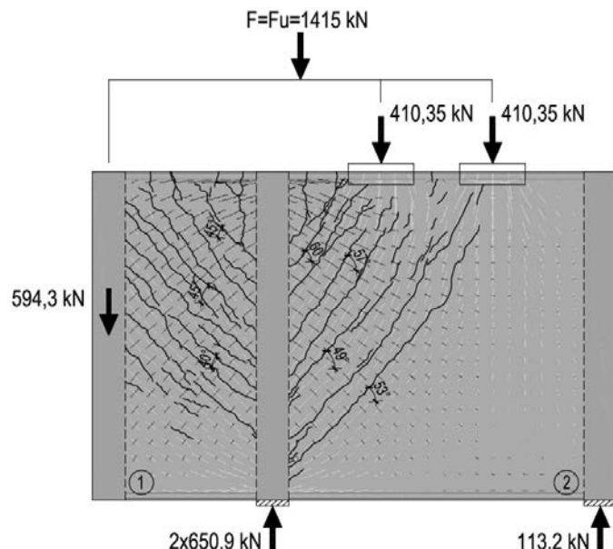
Rys. 11. Obraz zarysowania tarczy DB-II na tle trajektorii naprężeń głównych, przy sile niszczącej wspornik F_u = 1415 kN
