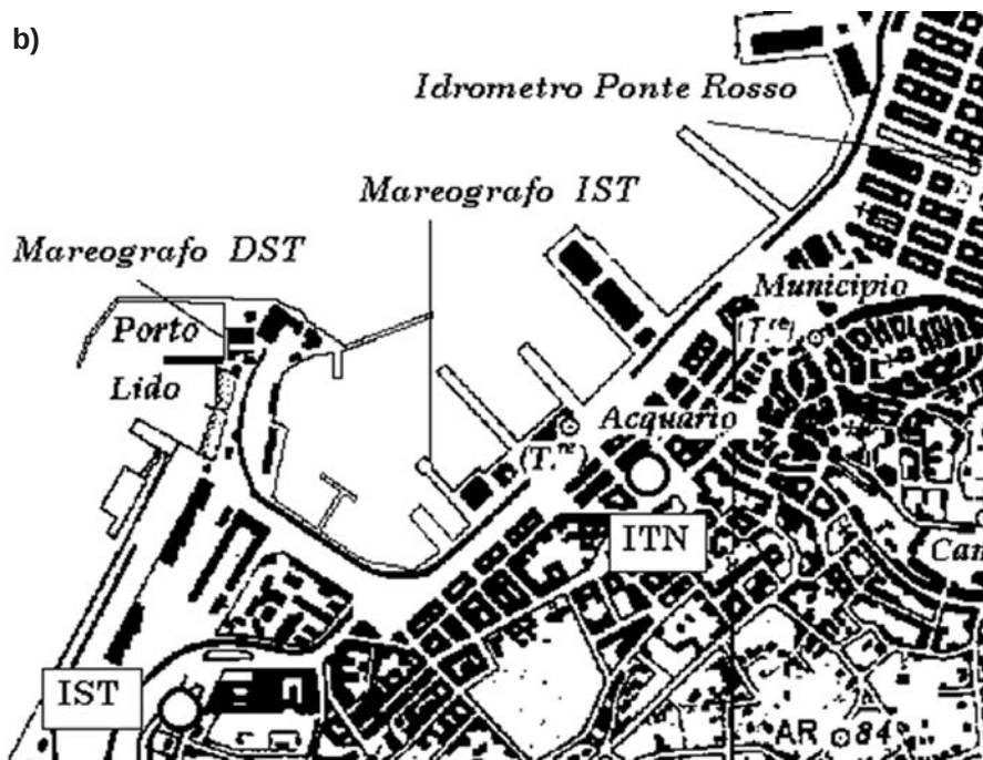
Rys. 9. Lokalizacja stacji mareograficznej Triest: położenie stacji w Zatoce Triesteńskiej Morza Adriatyckiego (a), usytuowanie stacji w porcie na moście Sartorio – Mareografo IST (b) [26]
