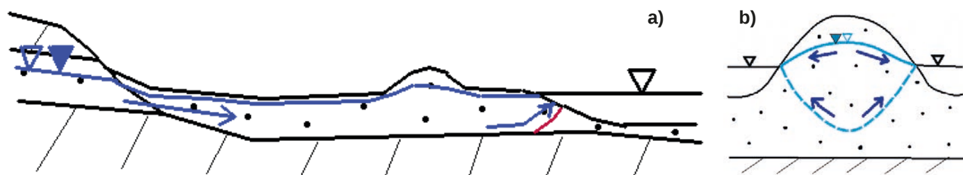
Rys. 5. Schemat warunków hydrogeologicznych wybrzeża płaskiego: a) niziny nadmorskie, b) mierzeje
