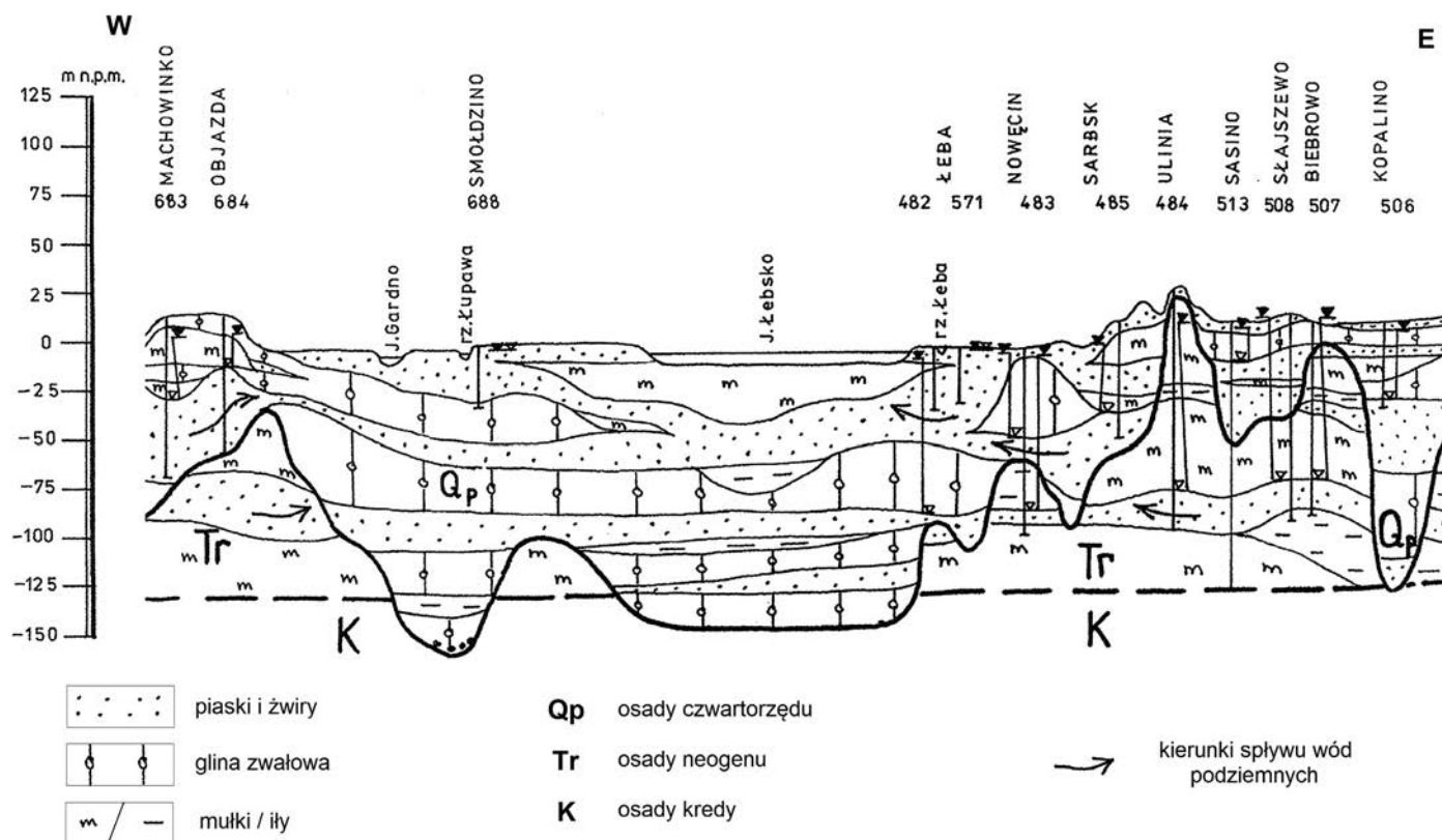
Rys. 4. Przekrój hydrogeologiczny przez fragment wybrzeża płaskiego
