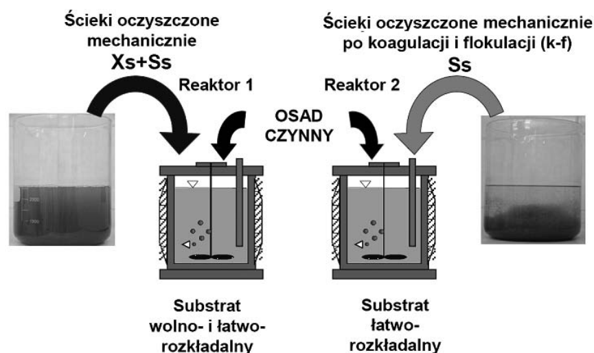
Rys. 1. Schemat przedstawiający procedurę badawczą oceny wpływu X_s na kinetykę procesów biochemicznych z użyciem równoległych reaktorów nieprzepływowych
