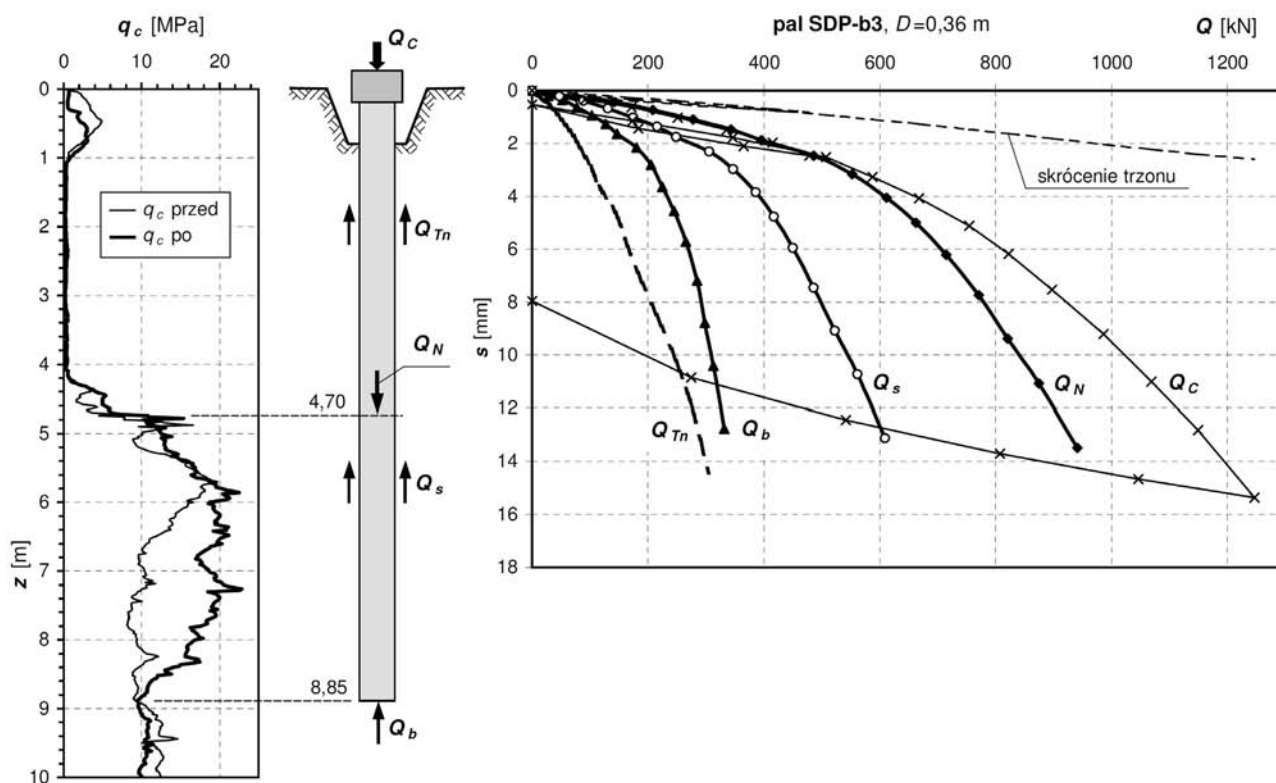
Rys. 2. Wyniki badania nośności pala SDP-b3 z rozdziałem obciążenia na opory gruntu wzdłuż pobocznic i pod podstawą pala
