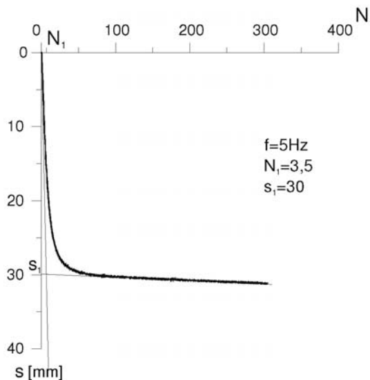
Rys. 4. Przebieg procesu tonięcia płytki w warstwie nawodnionego gruntu
