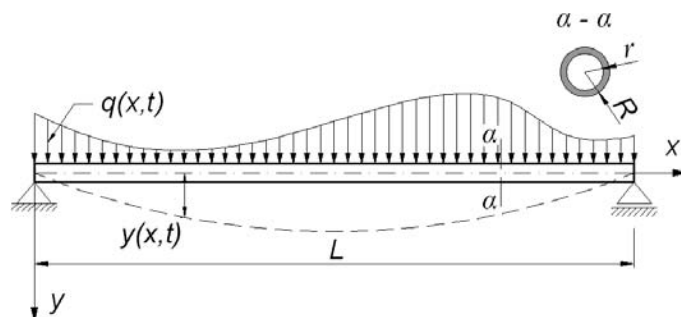
Rys. 1. Pojedyncze prześło rurociągu
