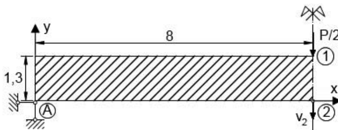
Rys. 2. Geometria tarczy z warunkami brzegowymi oraz obciążeniem
