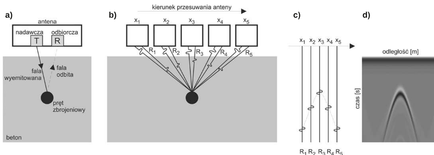
Rys. 1. Schemat działania metody georadarowej
