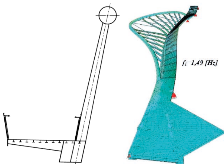
Rys. 5. Przekrój poprzeczny przez przęsło łukowe – wersja zmodyfikowana projektu
