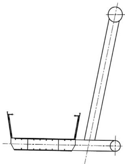
Rys. 2. Przekrój poprzeczny przez przęsło łukowe – wersja pierwotna projektu
