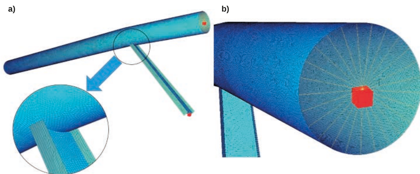
Rys. 7. Wizualizacja modelu obliczeniowego (W14) wersja pierwotna a) widok ogólny i szczegółowy modelu, b) sztywne elementy belkowe łączące krawędzie elementów powłokowych z punktem brzegowym
