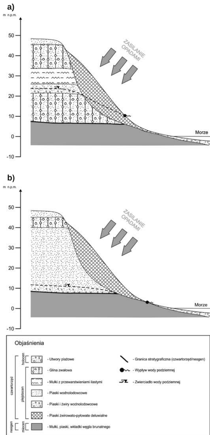
Rys. 2. Schematy zasilania badanych wypływów w obrębie terenu badań a) obszar na zachód od Lebskiego Żlebu, b) obszar na wschód od Lebskiego Żlebu
