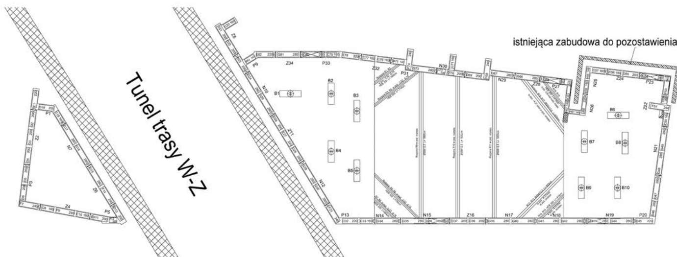
Rys. 4. Rzut ścian szczelinowych. Budynek biurowo-usługowy przy ul. Senatorskiej w Warszawie [27]
