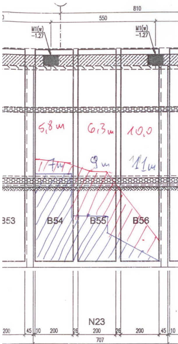
Rys. 2. Brak możliwości wykonania dolnej części ściany szczelinowej ze względu na występujące w podłożu glazy [4]
