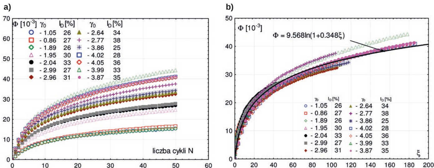
Rys. 1. Zagęszczenie gruntu niespoistego poddanego cyklicznemu prostemu ścinaniu przy różnych wartościach amplitudy odkształcenia postaciowego (a), uniwersalna krzywa zagęszczania (b)
