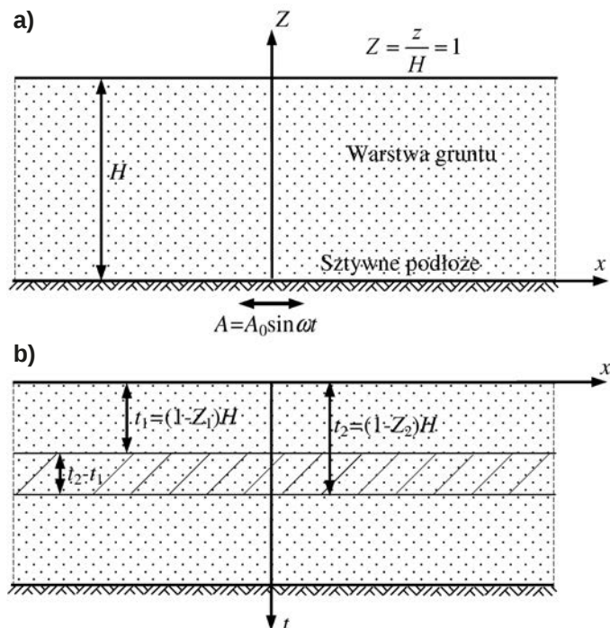
Rys. 2. Warstwa gruntu na sztywnym podłożu
