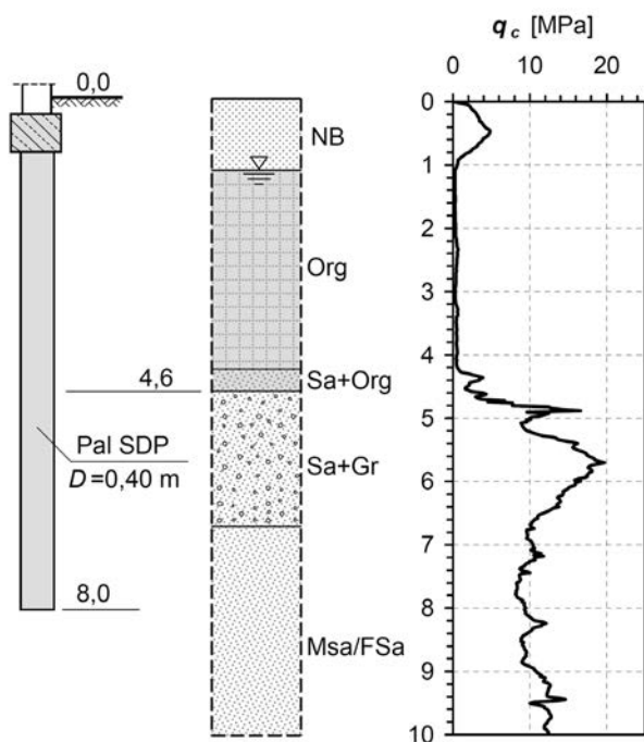
Rys. 3. Przyjęty profil geotechniczny do przykładu nr 1
