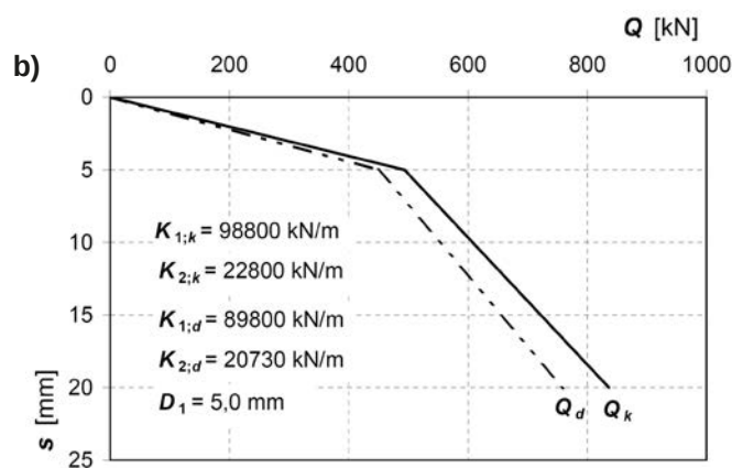
Rys. 4. Charakterystyki obciążenie – osiadanie pala SDP
