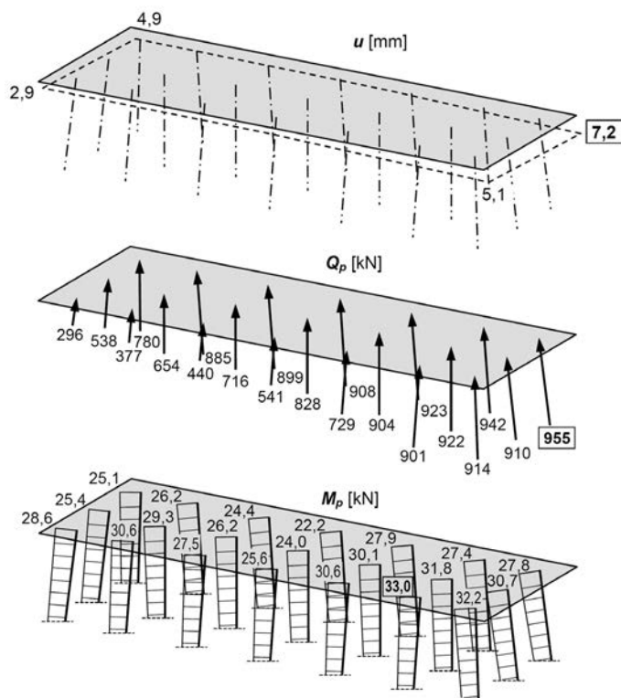
Rys. 9. Wyniki obliczeń do przykładu nr 2
