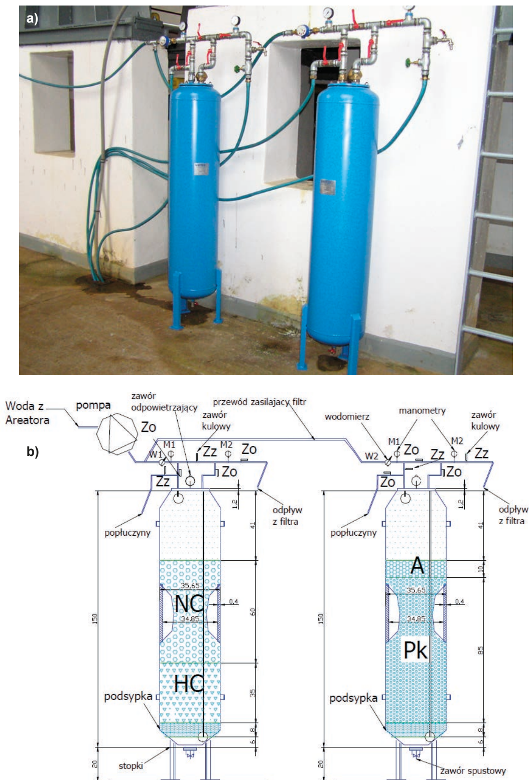
Rys. 3. Stacja pilotowa a) widok stanowiska badań technologicznych, b) schemat [7]
