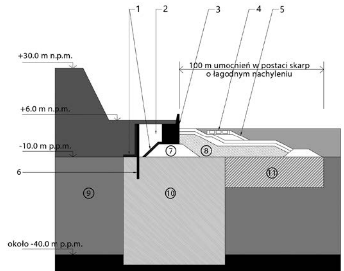
Rys. 2. Przekrój przez obrzeże wysypiska wybudowanego metodą kesonową, z zastosowaniem palowania zaporowego ( triple tubular steel pile method ). 1 – izolacja przeciwwodna, 2 – wypełnienie zmieszonym materiałem, 3 – keson, 4 – basen pływowy, 5 – skały oporowe, 6 – osłona z pali stalowych, 7 – wał z gruzu, 8 – podbudowa z piasku, 9 – dno zatoki – grunt spoisty, 10 – grunt stabilizowany włąębnie cementem (CDM – cement deep mixing ), 11 – piaski zagęszczane za pomocą pali (SCP – sand compaction pile method ) Opracowanie własne na podstawie [7]
