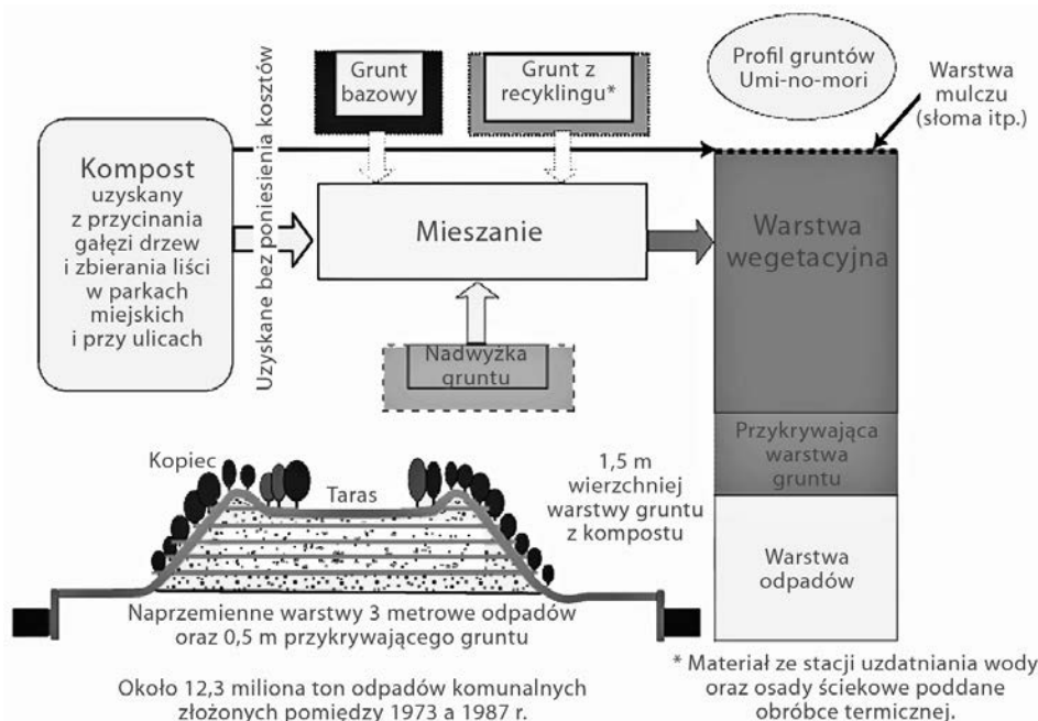
Rys. 3. Schemat mieszanki tworzącej warstwę wegetacyjną na Sea Forest Island [8]
