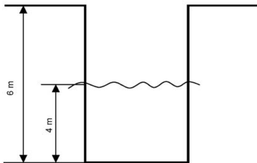
Rys. 8. Cechowanie studzienki zgodnie z normą PN-EN13598: mniejsza wartość określa maksymalną głębokość wód gruntowych powyżej dna kanału przełotowego, większa – maksymalną głębokość instalacji studzienki
