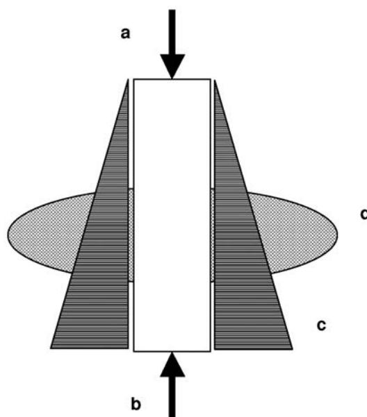
Rys. 2. Charakterystyczne obciążenia działające na kanalizacyjną studzienkę rewizyjną a – zewnętrzne (w tym dynamiczne od transportu), b – siła wyporu nawodnionego podłoża, c – od podłoża, d – dodatkowo od okresowo pęczniejącego podłoża
