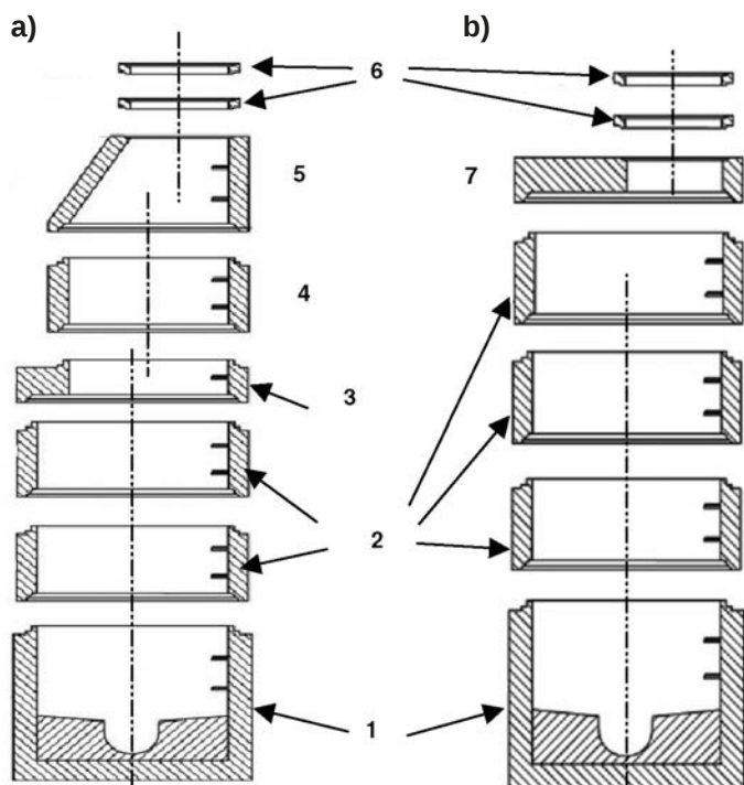
Rys. 7. Podstawowe odmiany betonowych kanalizacyjnych studzienek rewizyjnych ze zwężką redukcyjną (a) i z płytą pokrywową (b) 1 – dno studni z kinetą, 2 – kręgi betonowe, 3 – płyta redukcyjna, 4 – krąg komina, 5 – zwężka redukcyjna, 6 – pierścień dystansowy, 7 – płyta pokrywowa; na podstawie [3]
