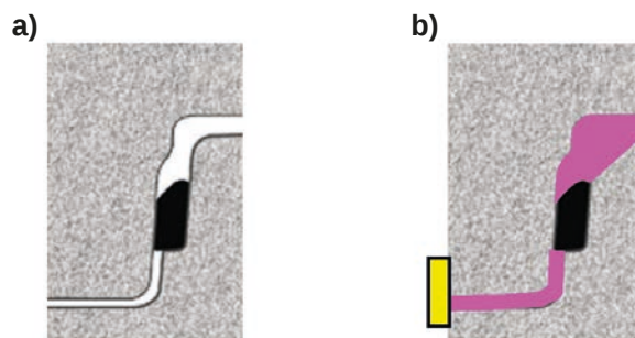
Rys. 4. Zwanie elementów betonowych łączonych na uszczelkę a) pod wpływem masy własnej kręgów powyżej złącza, b) z dodatkowym doszczelnieniem specjalną masą
