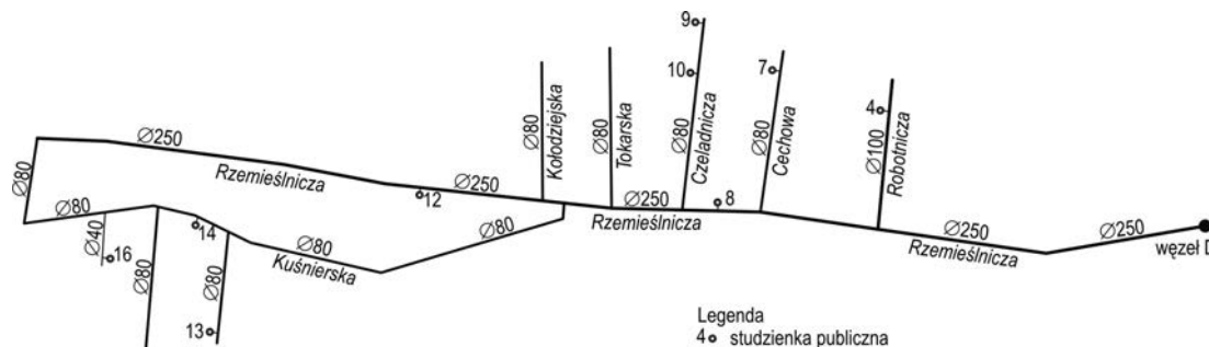
Rys. 11. Projekt planu wodociągu dla Nowego Obłuża
