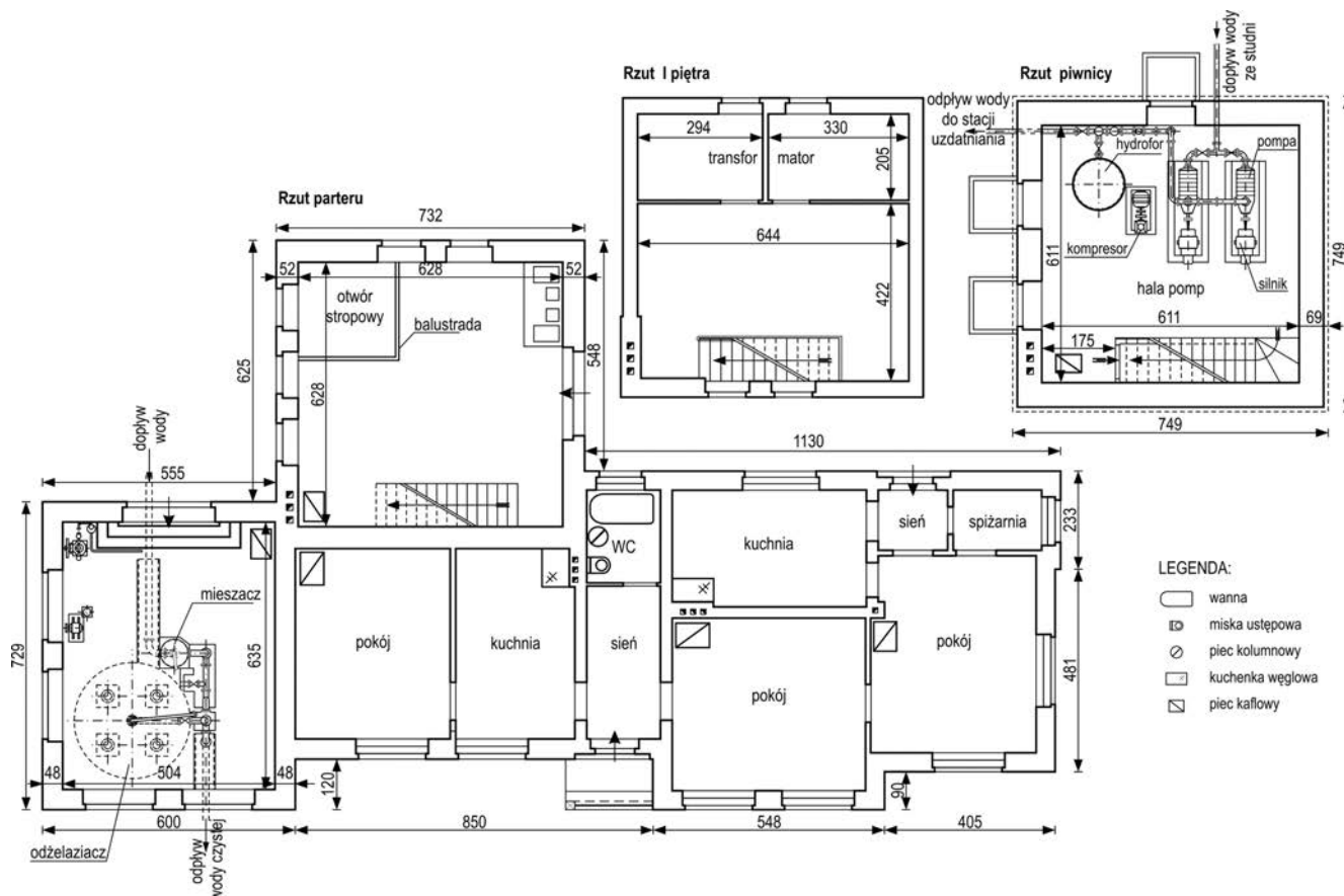
Rys. 3. Rzuty kondygnacji budynku hali pomp, stacji uzdatniania i mieszkań na ujęciu „Oksywie” (opracowanie własne na podstawie materiałów archiwalnych AP Gdyni. 768/28)
