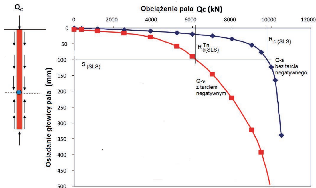
Rys. 5. Przykładowe próbne obciążenie pala o średnicy 1,0 m z tarcieniem negatywnym i bez tarcia negatywnego [6]
