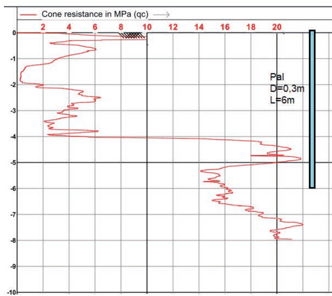
Rys. 4. Sondowanie CPT4
