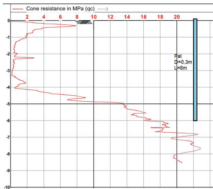
Rys. 2. Sondowanie CPT2
