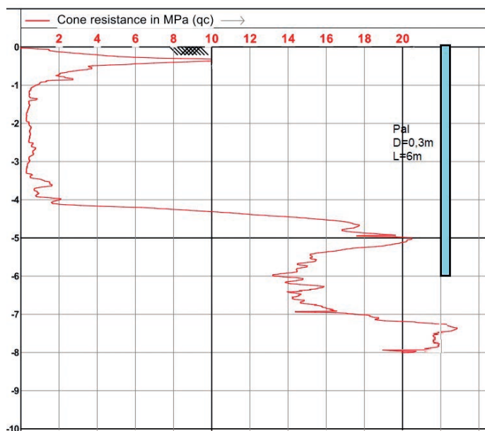
Rys. 1. Sondowanie CPT1
