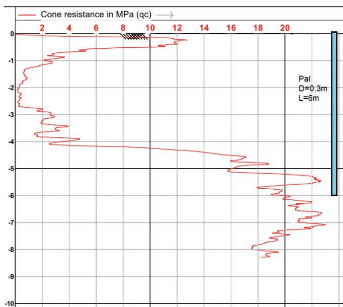
Rys. 3. Sondowanie CPT3
